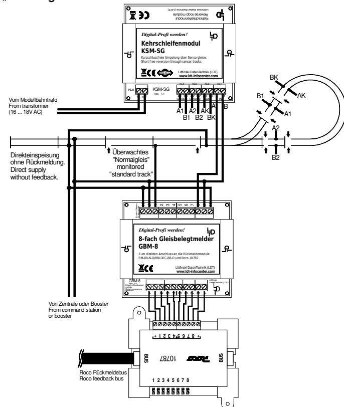
Abbildung 3: Über den Ausgang 8 des GBM-8 wird über das Kehrschleifenmodul KSM-SG die Kehrschleife inkl. der Sensorgleise überwacht. Ausgang 1 überwacht ein „Normalgleis“.
